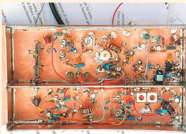
Bovenaanzicht van de BITX20
